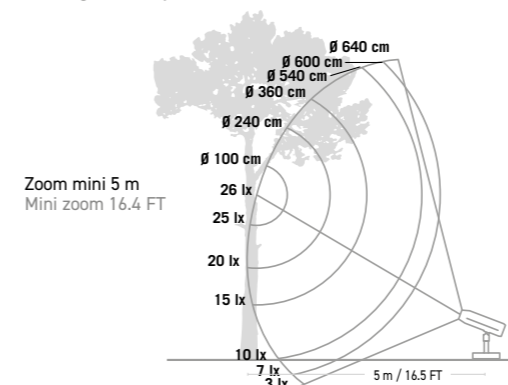
LUX /DISTANCE pour une implantation à 5 m LUX /DISTANCE form a position 16.4 FT away
