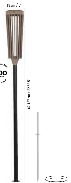
TORCHE TECKA® À PLANTER OU À SCELLER 2 HAUTEURS AJUSTABLES TECKA GARDEN TORCH TO PLANT, TWO ADJUSTABLE HEIGHTS
