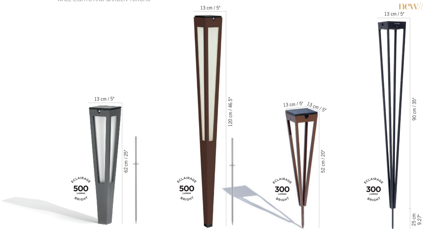
APPLIQUE / TORCHE TINKA® Livrée avec pic à planter en inox TINKA® mini torch delivered with inox spike to plant.
