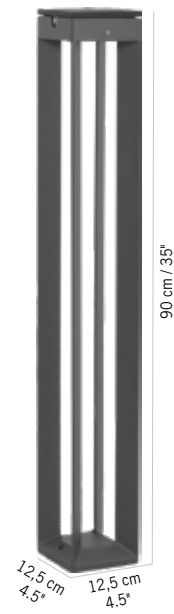
BORNE BLADE À FIXER BLADE pathway light to fix
