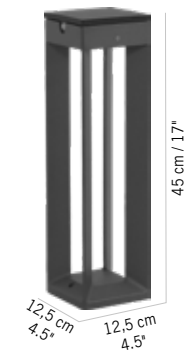
BORNE BLADE À FIXER BLADE pathway light to fix
