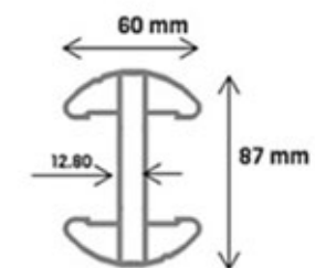
Vue en coupe EXPERT PLUS (450A)
