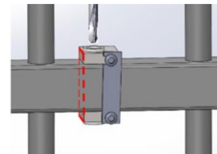
L'outil facilite les opérations : le perçage est guidé et la découpe des lisses est parfaitement droite.
