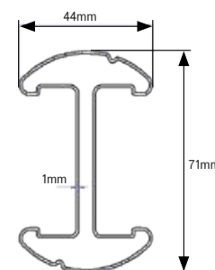
Vue de coupe du poteau EXPERT (260S)
