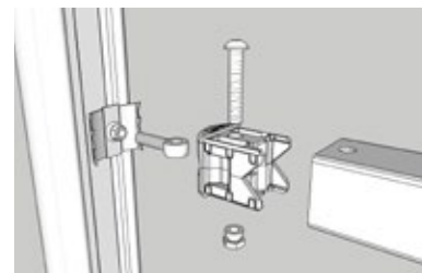
Eclaté du système de fixation du barreaudage TIVANO au poteau EXPERT
