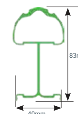
Coupe du poteau EXPERT (250A)
